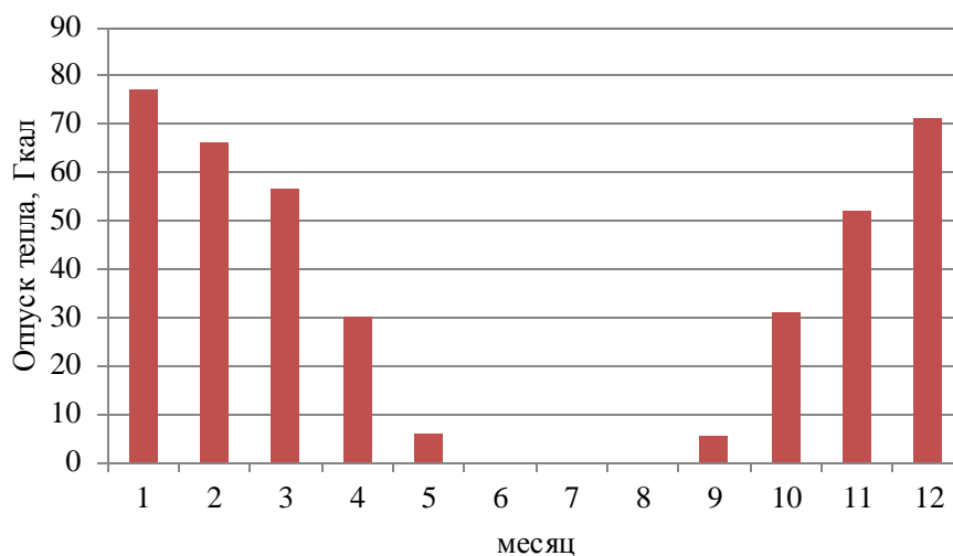
Рис. 3 – Оптимальный температурный график отпуски тепловой энергии для котельной п. Берегаево
