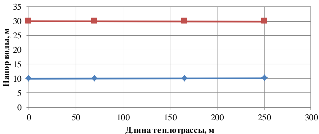
Рис. 5 – Пьезометрический график тепловой сети котельной п. Берегаево
